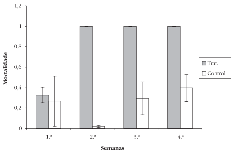
Figura 4 – Percentagem de mortalidade observada nos sacos de plástico expostos ao sol e nos sacos de controlo.
